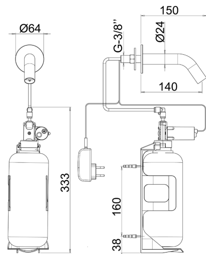
Version travers cloison, sur secteur, RES-641-S1
