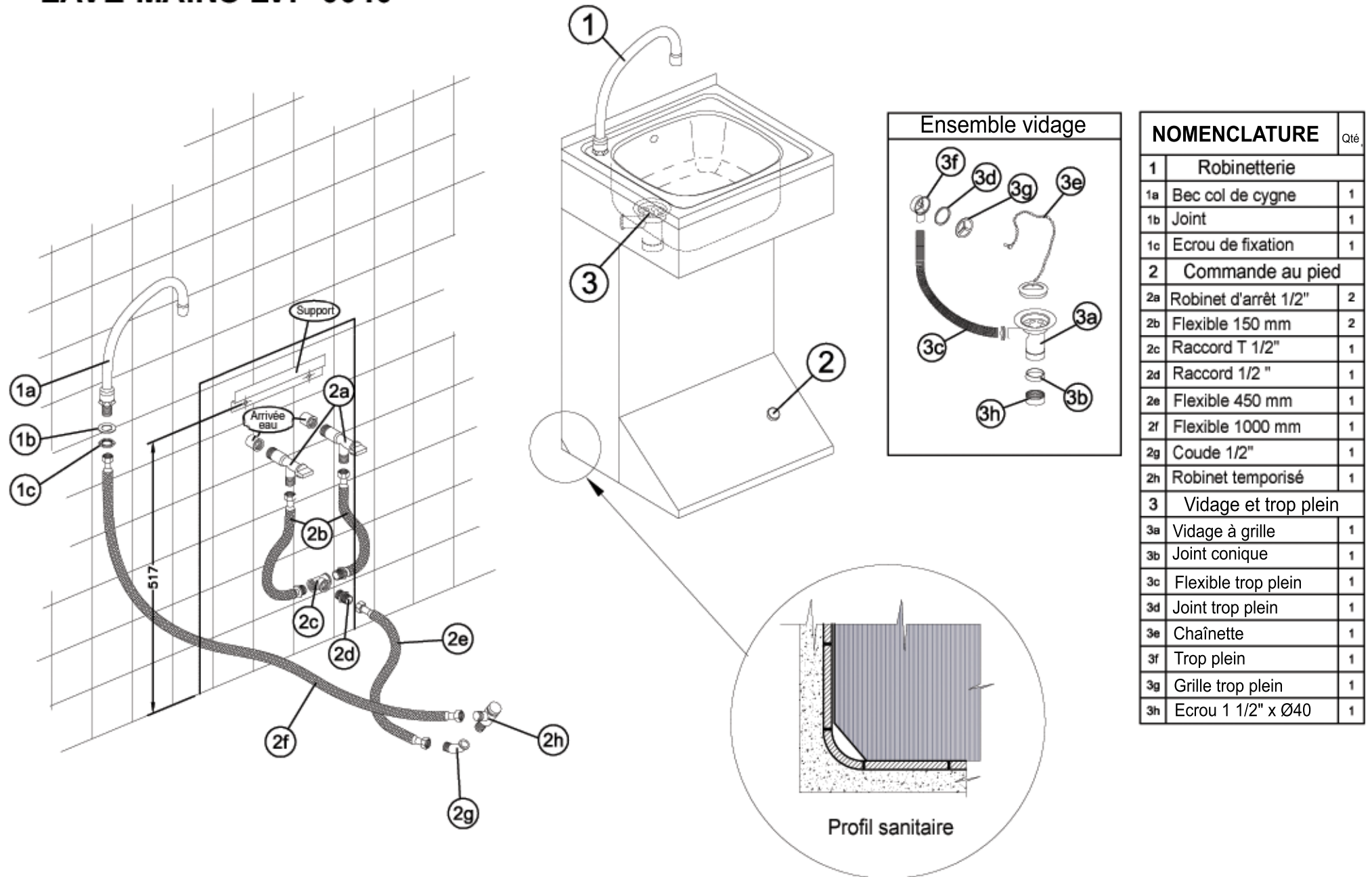
SCHEMA DE L'INSTALLATION
