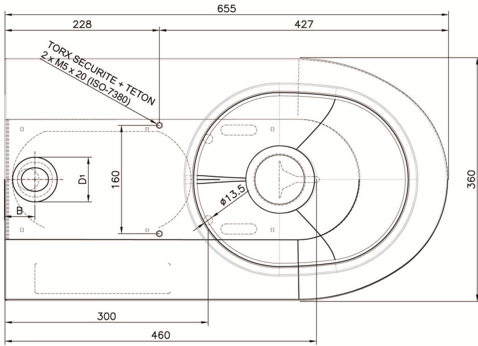
WC inox à poser ULTIMA alimentation verticale apparente réf. IN-005-AV
